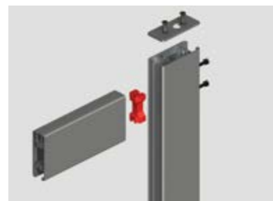
Assemblage mécanique
